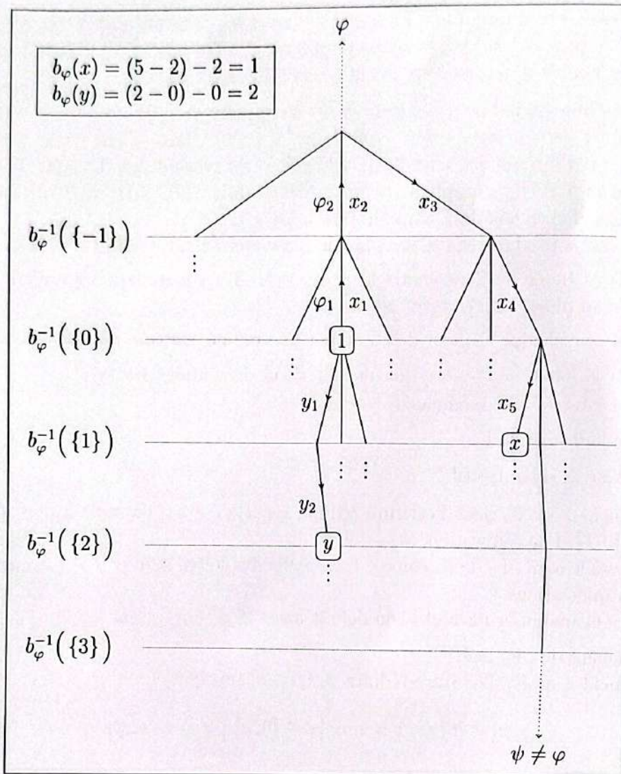
FIGURE 2 - Lignes de niveau de la fonction b_\varphi
