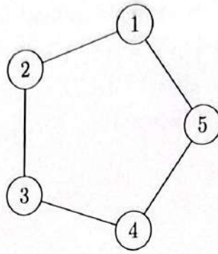
FIGURE 1 – Graphe cyclique à 5 sommets
